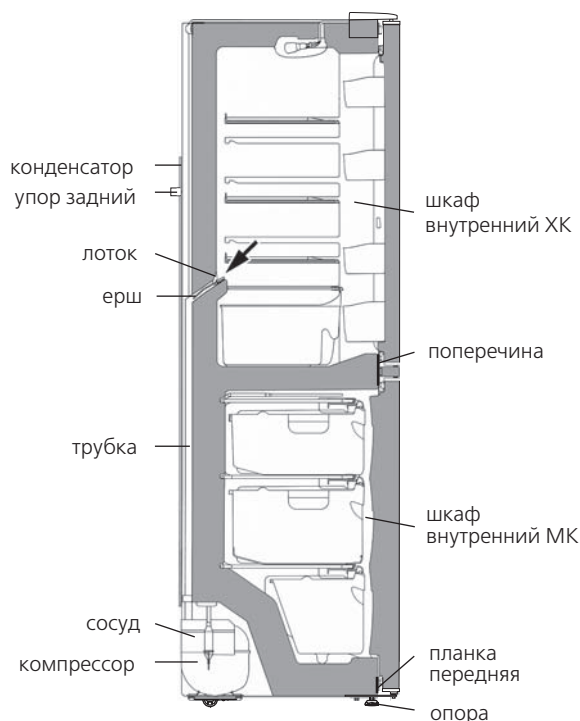
Рисунок 9 — Схема слива талой воды
